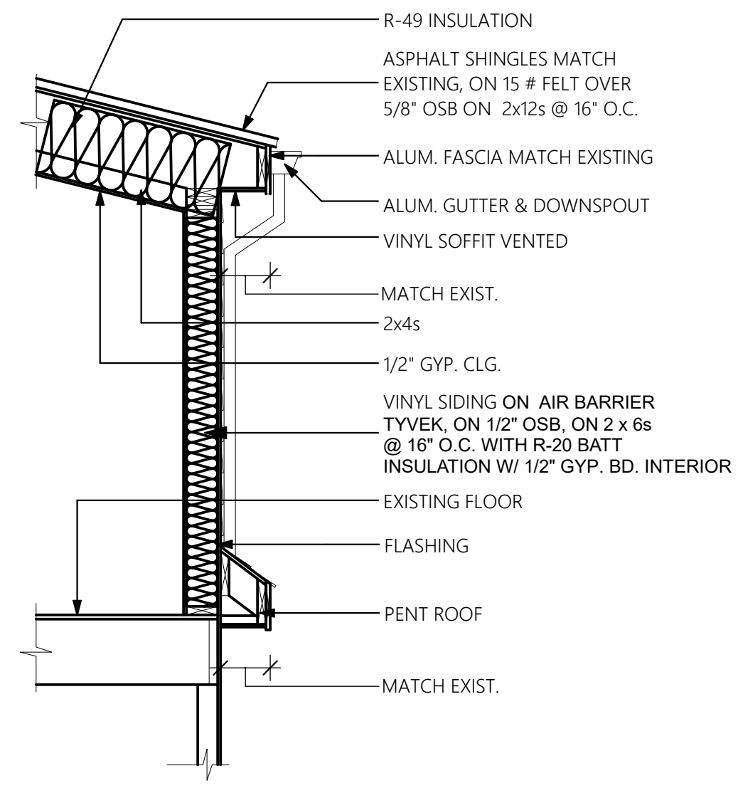
4 A-2 DETAIL SCALE: 1/2" = 1'-0"
